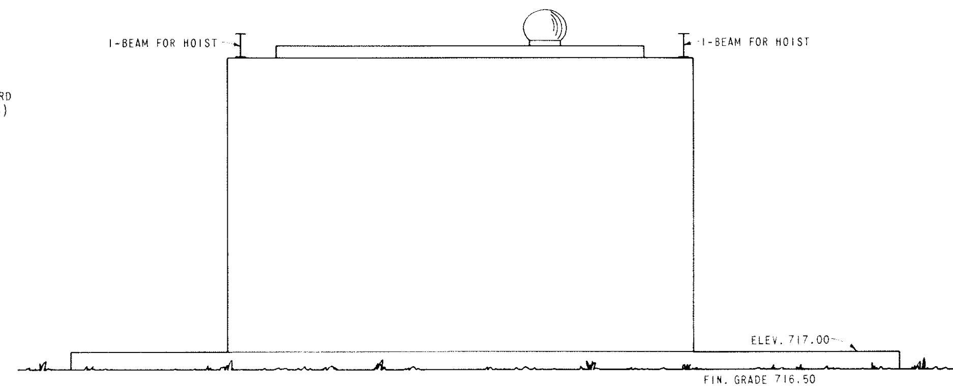
WEST ELEVATION SCALE: 1/2" = 1'-0"
