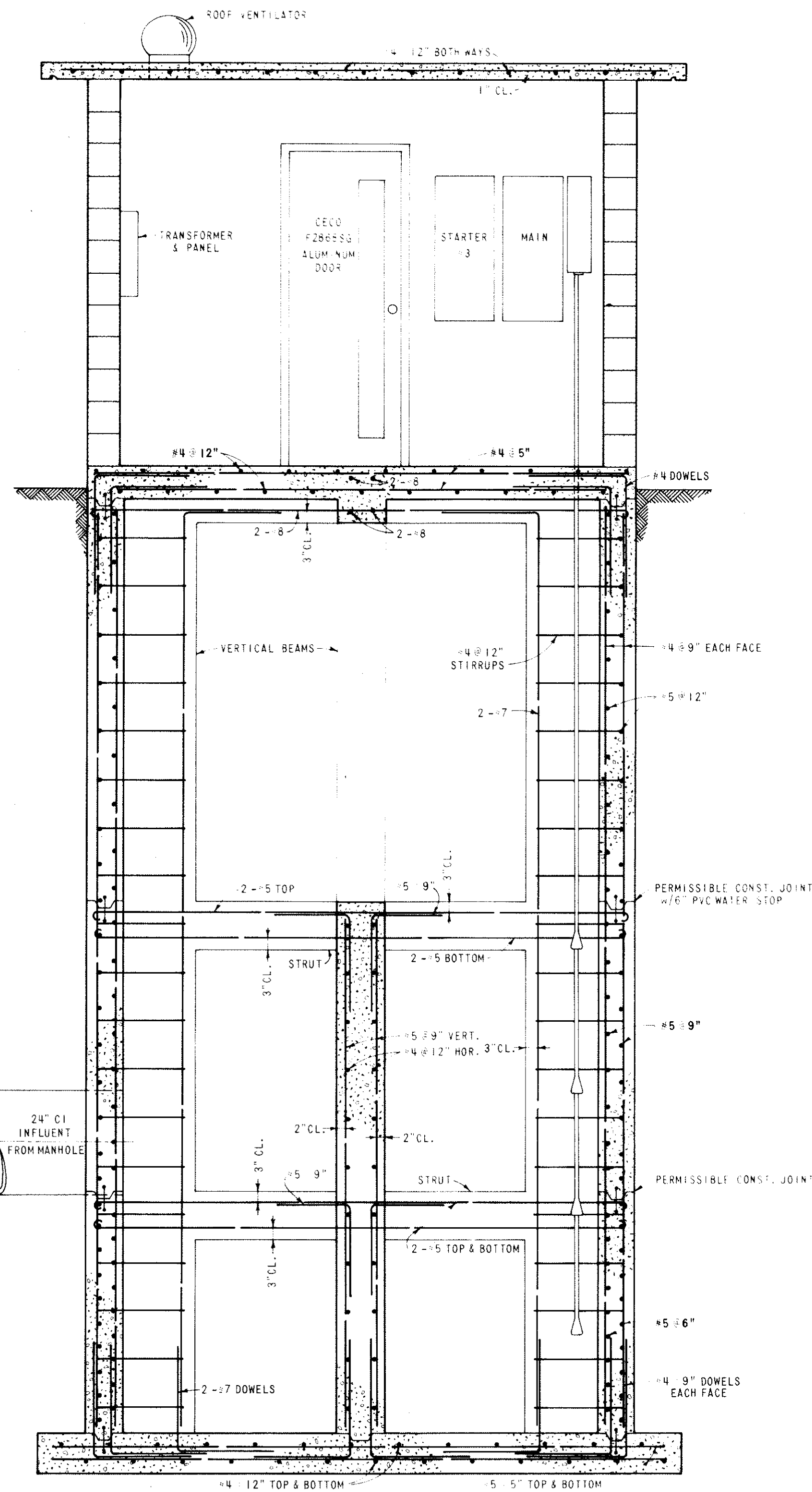
SECTION B-B SCALE: 1/2" = 1'-0"
